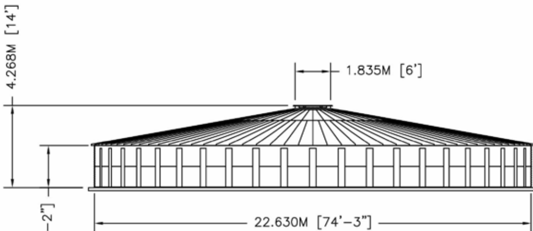
ELEVATION
